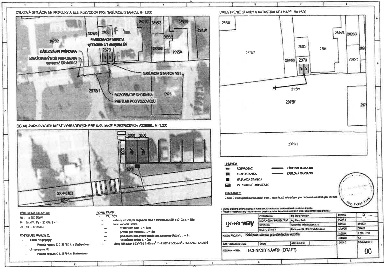
Príloha č.1: Celková situácia stavby „Nabíjacia stanica pre elektrické vozidlá – Tesco Sládkovičovo“
